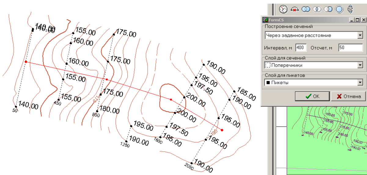
Рисунок 7.2. Построение поперечных сечений
