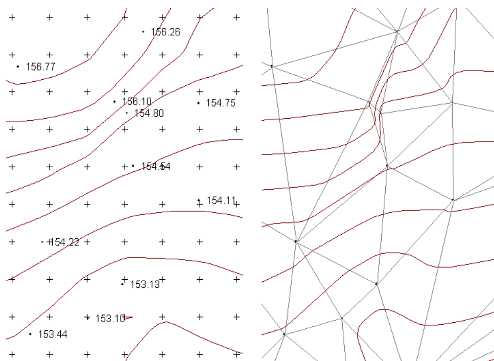
Рисунок 10.1. Фрагменты ЦМР и TIN
