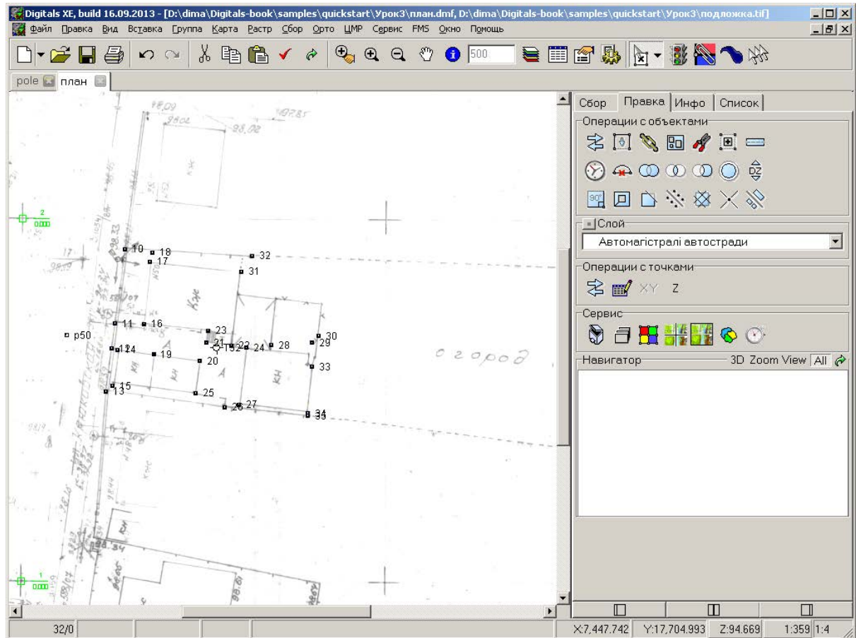
Рисунок 3.4. Пример полевой съемки с растровой подложкой
