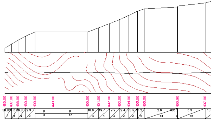
Рисунок 10.3. Фрагмент профиля
